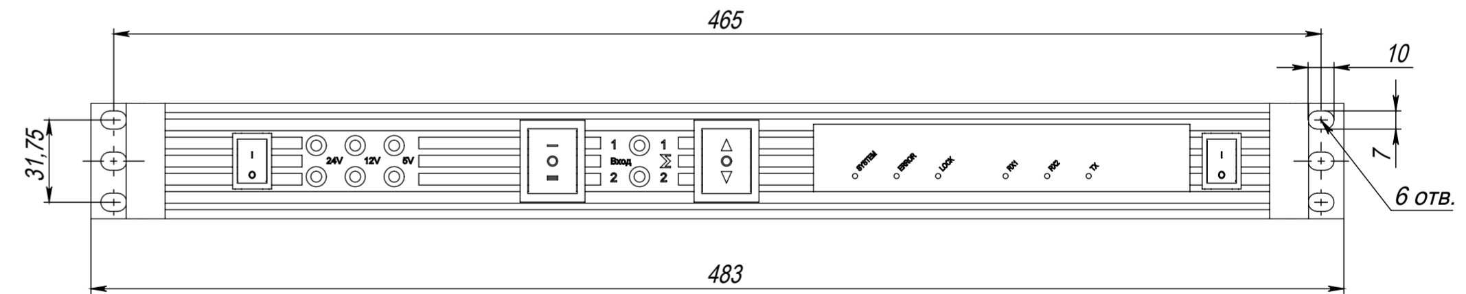
Спутниковый маршрутизатор UHP-200
