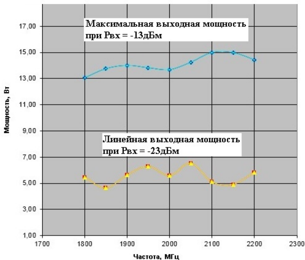
АЧХ блока УМ1821-12
